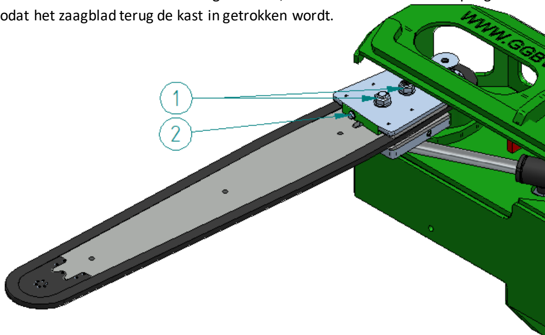
Wisselinrichting zaagblad/ketting
